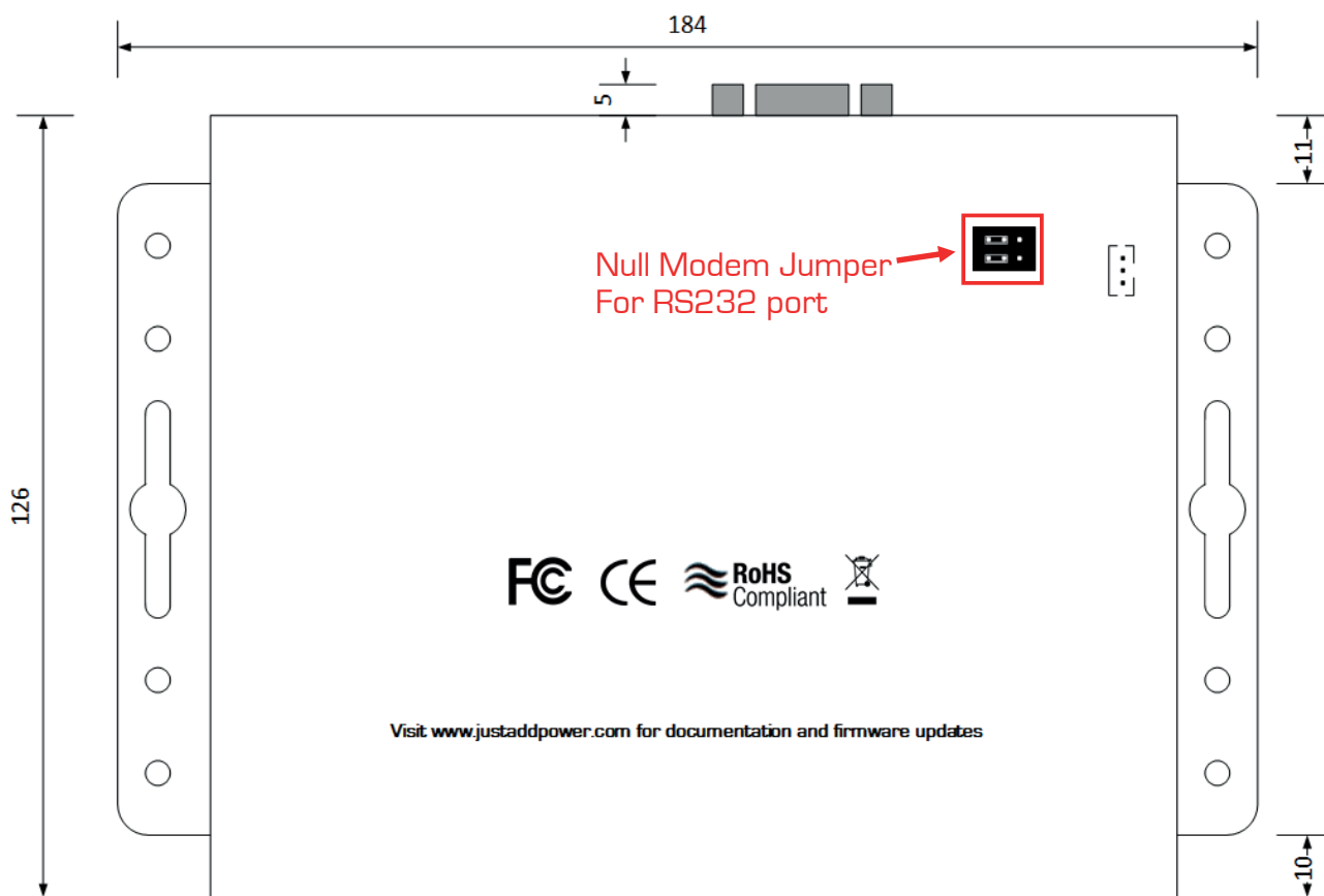
716VGA Bottom
